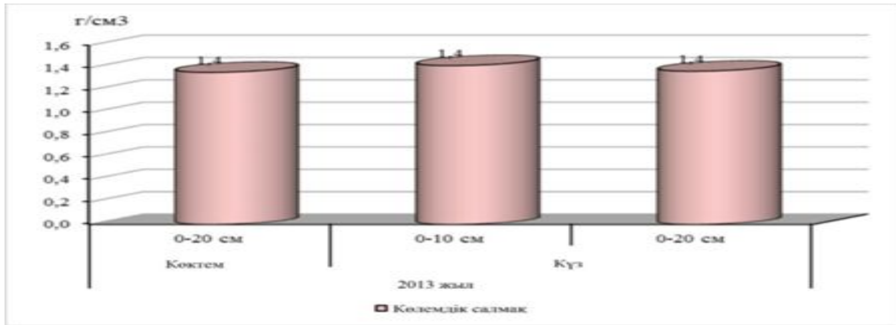
Сурет 9 – Топырақгрунттарының көлемдік салмағы
