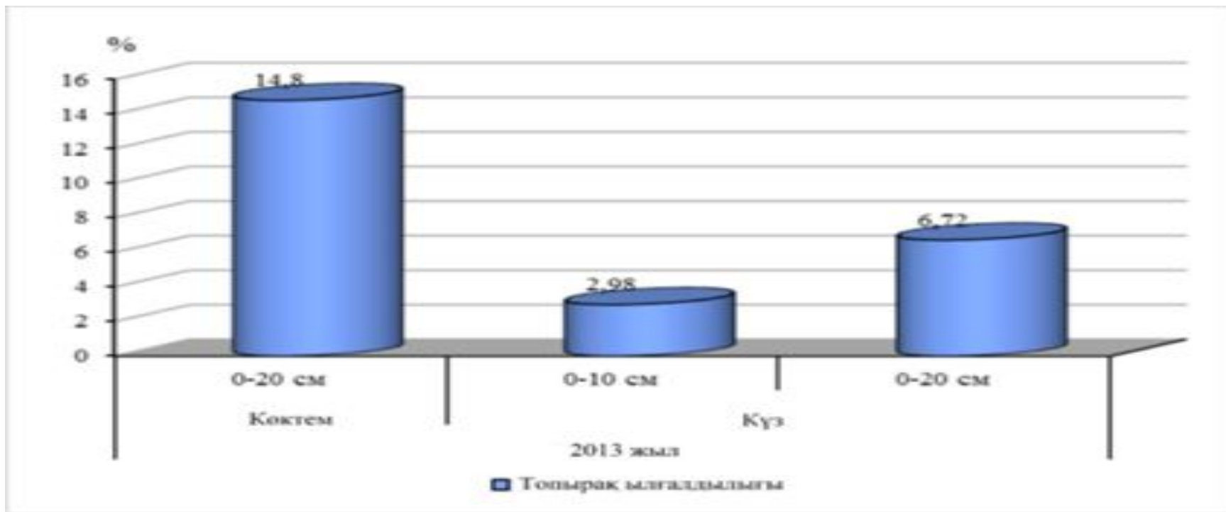
Сурет 8– Топырақгрунттарының ылғалдылығы
