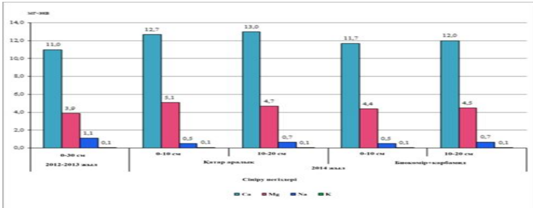
Сурет 7 – Тәжірибе теліміндегі топырақгрунттарының сіңіру негіздері
